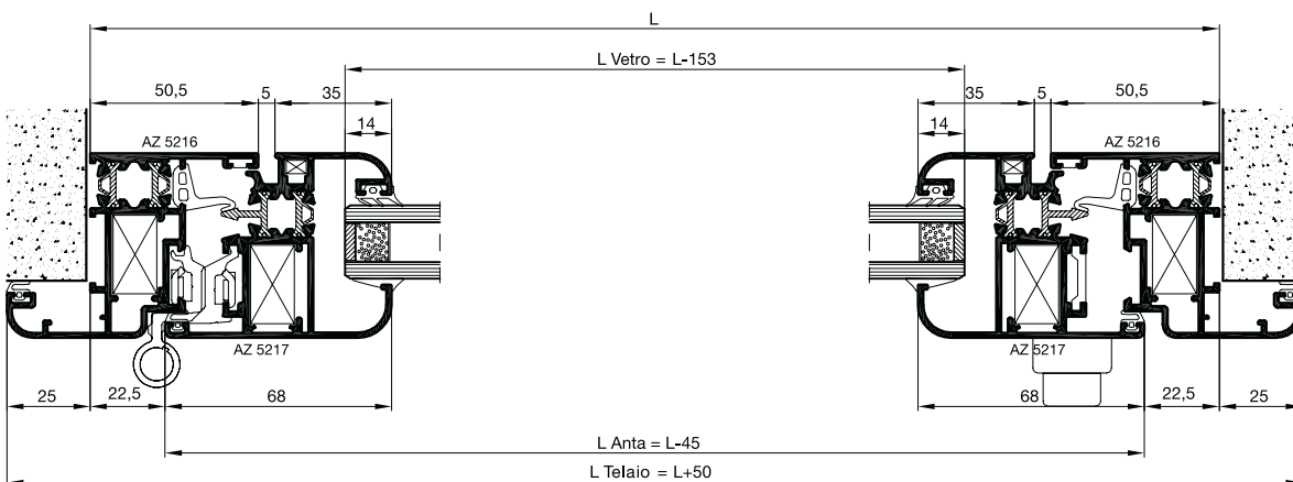
Sezione C-C'
