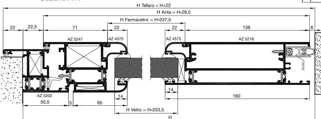
Sezione A-A'
