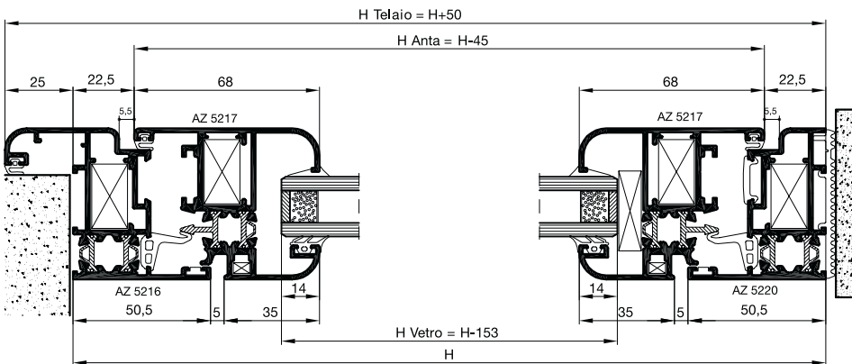
Sezione A-A'
