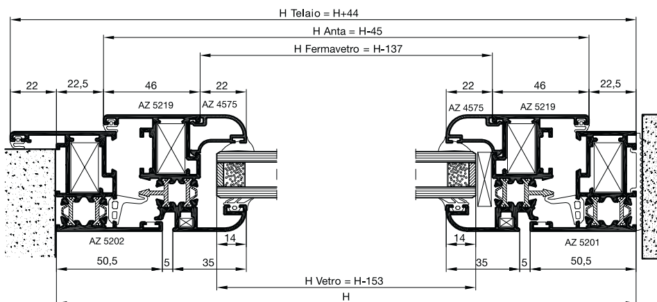
Sezione A-A'
