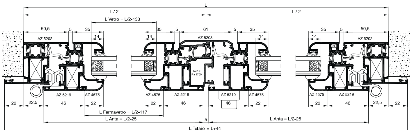
Sezione B-B'-B
