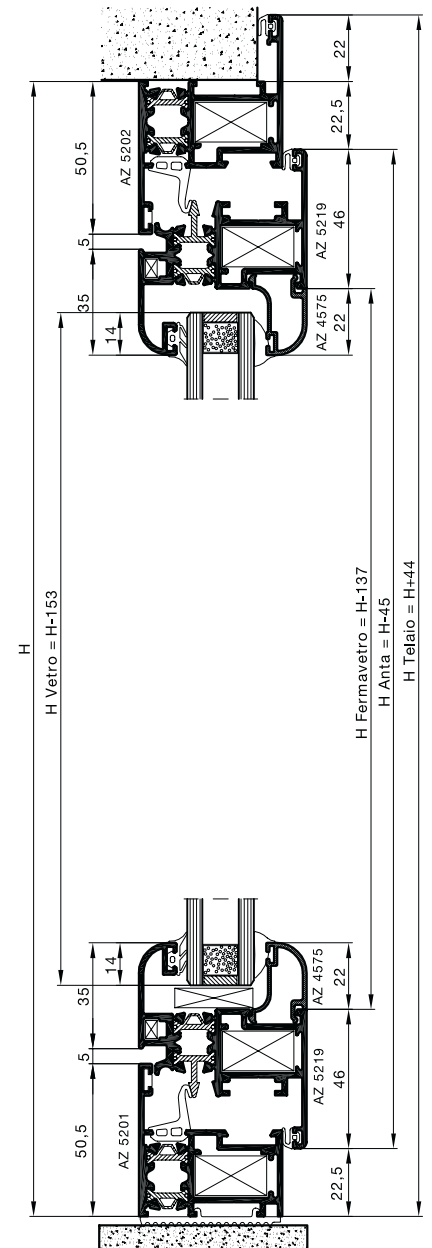
Sezione B-B'
