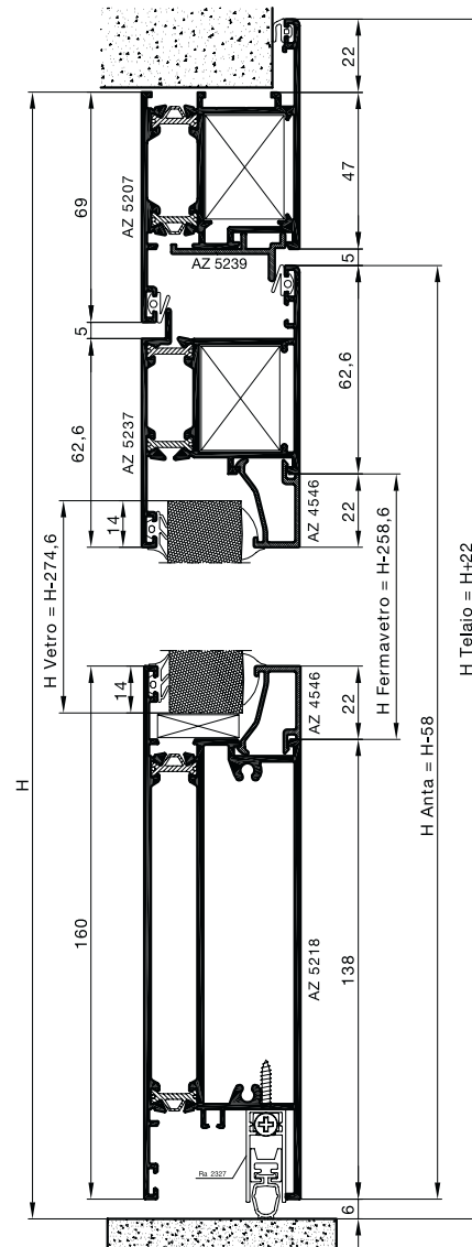
Sezione A-A'
