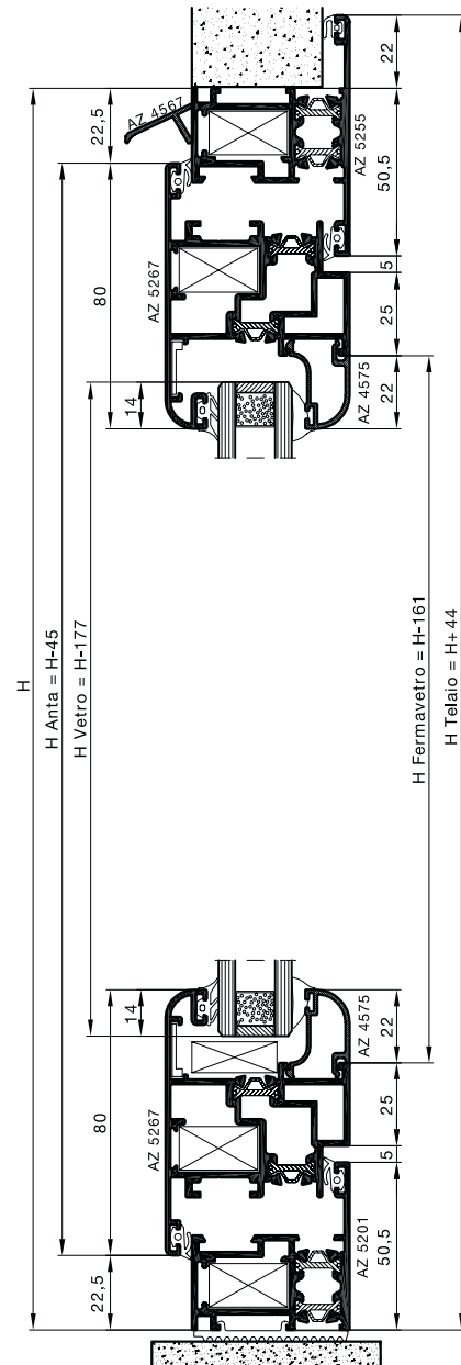
Sezione C-C'
