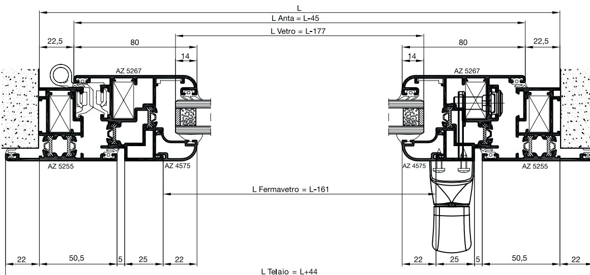
Sezione B-B'
