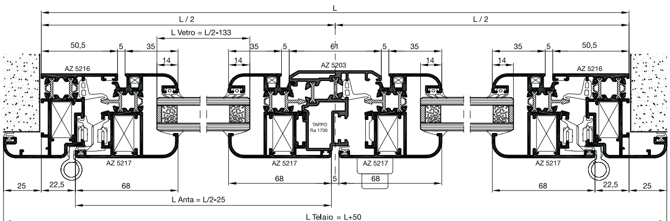
Sezione B-B'-B
