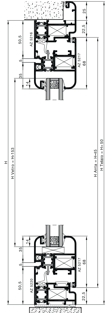
Sezione B-B'
