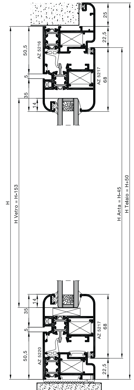
Sezione A-A'
